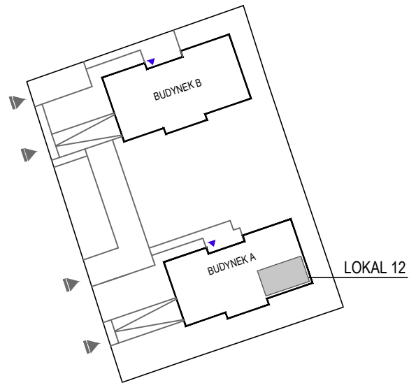
SCHEMAT RZUTU 2 PIĘTRA
